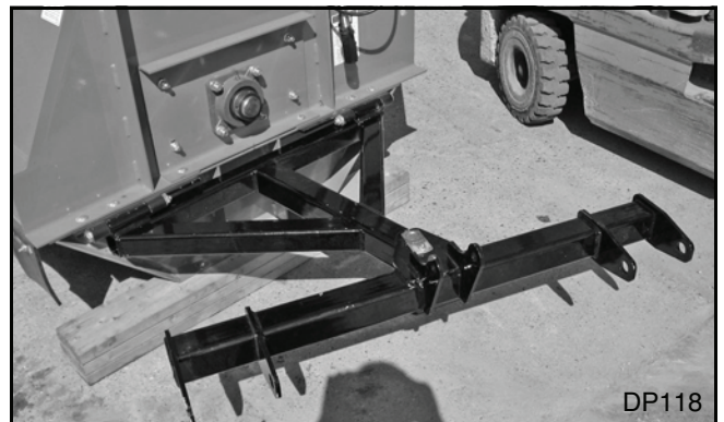
Figura 22. Reboque de extremidade - Engate rápido
