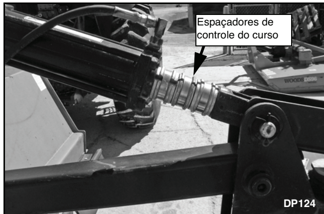
Figura 10. Ajuste da altura operacional
